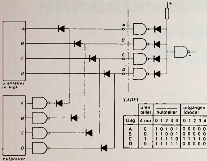
Fig. 2. Vergelijkingsprincipe.
